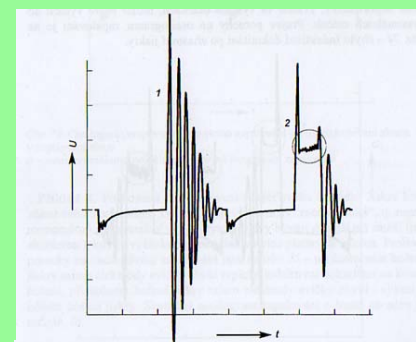
Obr. 72. Oscilogram nesprávně fungujícího zapalování 1 – v tomto válci nedošlo k zapálení, 2 – v tomto válci došlo ke správnému zapálení
